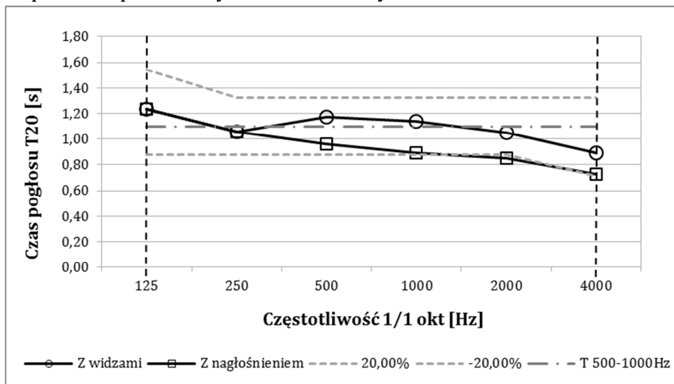
Rysunek 2 Czas pogłosu T_{20} w funkcji częstotliwości uzyskany na drodze symulacji obliczeniowej z zaznaczonym przedziałem dopuszczalnych odchyłek dla funkcji sali z i bez nagłośnienia. Wykresy dla sali z widzami.
